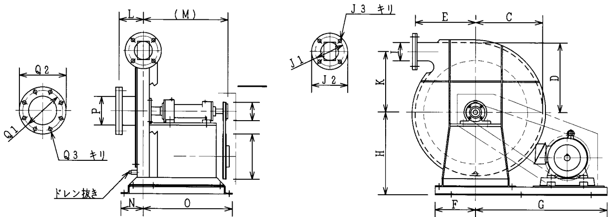
KES 28型寸法図
