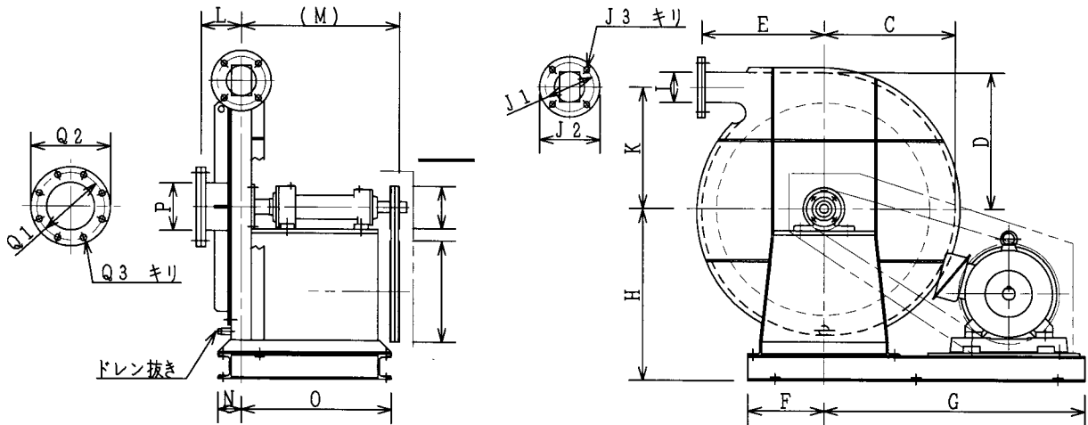
KES 48型寸法図
