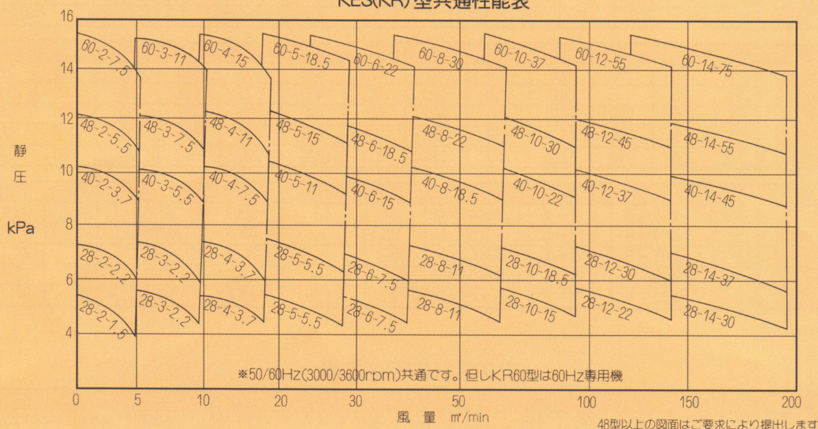
KES(KR)型共通性能表
