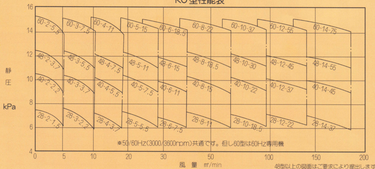
KO型性能表
